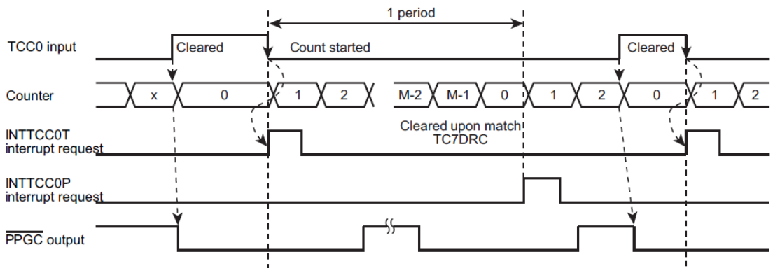
图 10.44 触发起始中断
