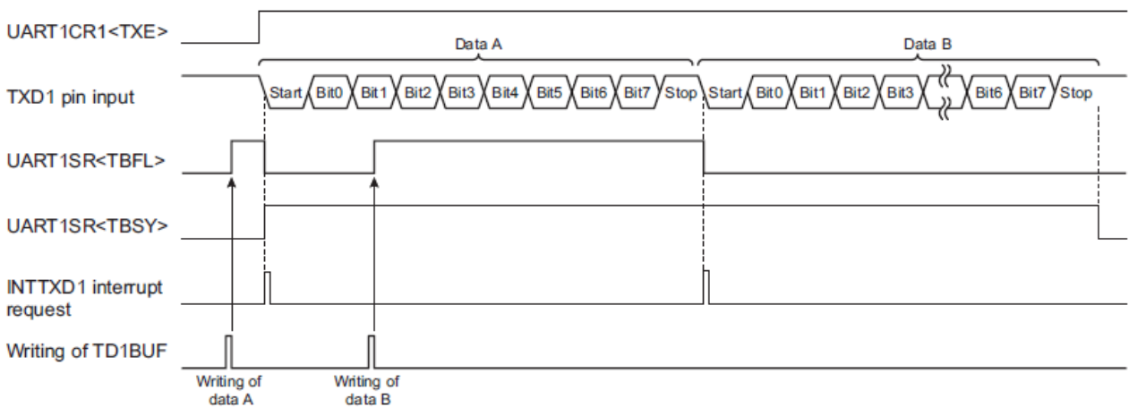
图 12.16 发送寄存器 已满的发生
