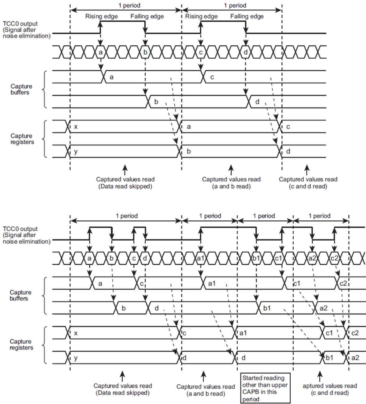
图 10.33 触发捕捉模式的操作范例
