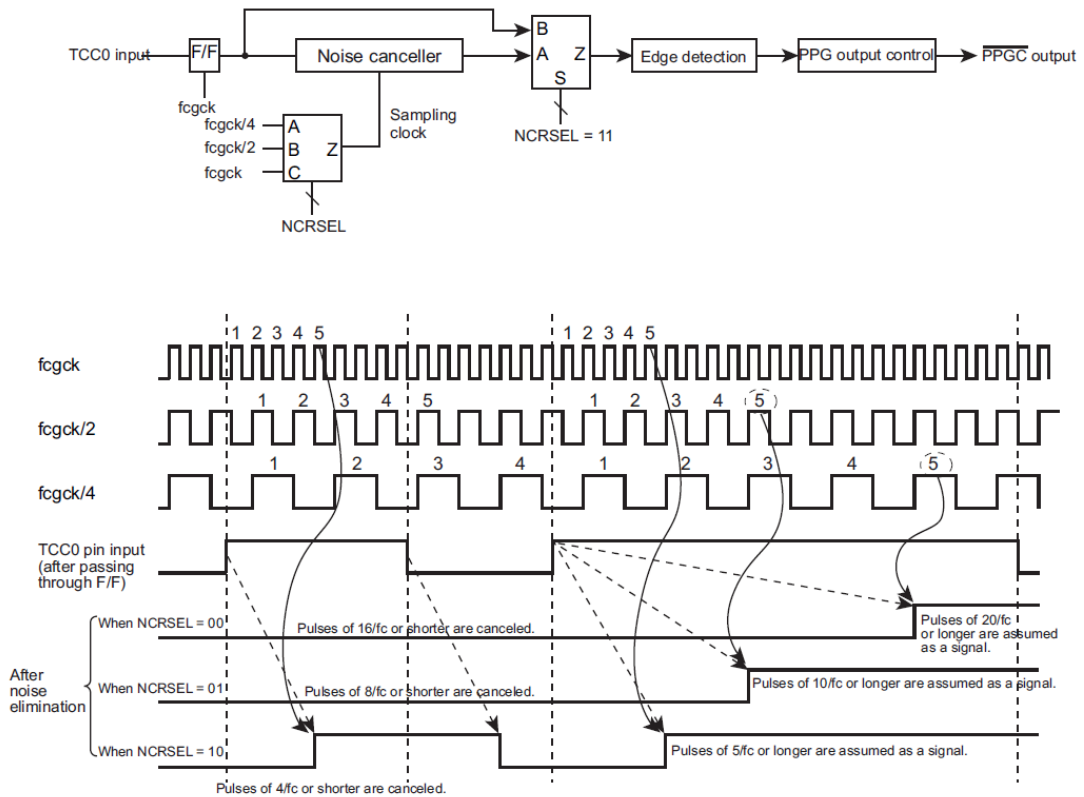
图 10.43 噪声消除
