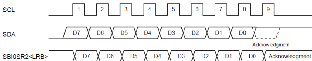
图 14.16 最后接收位变更监控
